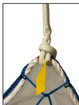
Opphengslinje m/løye SN 9001/ 9002 3m og 13,5 m
