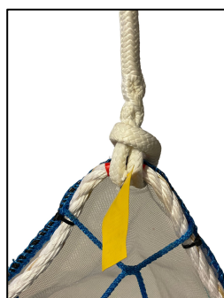
Opphengslinje m/øye SN 9001/ 9002 3m og 13,5 m
