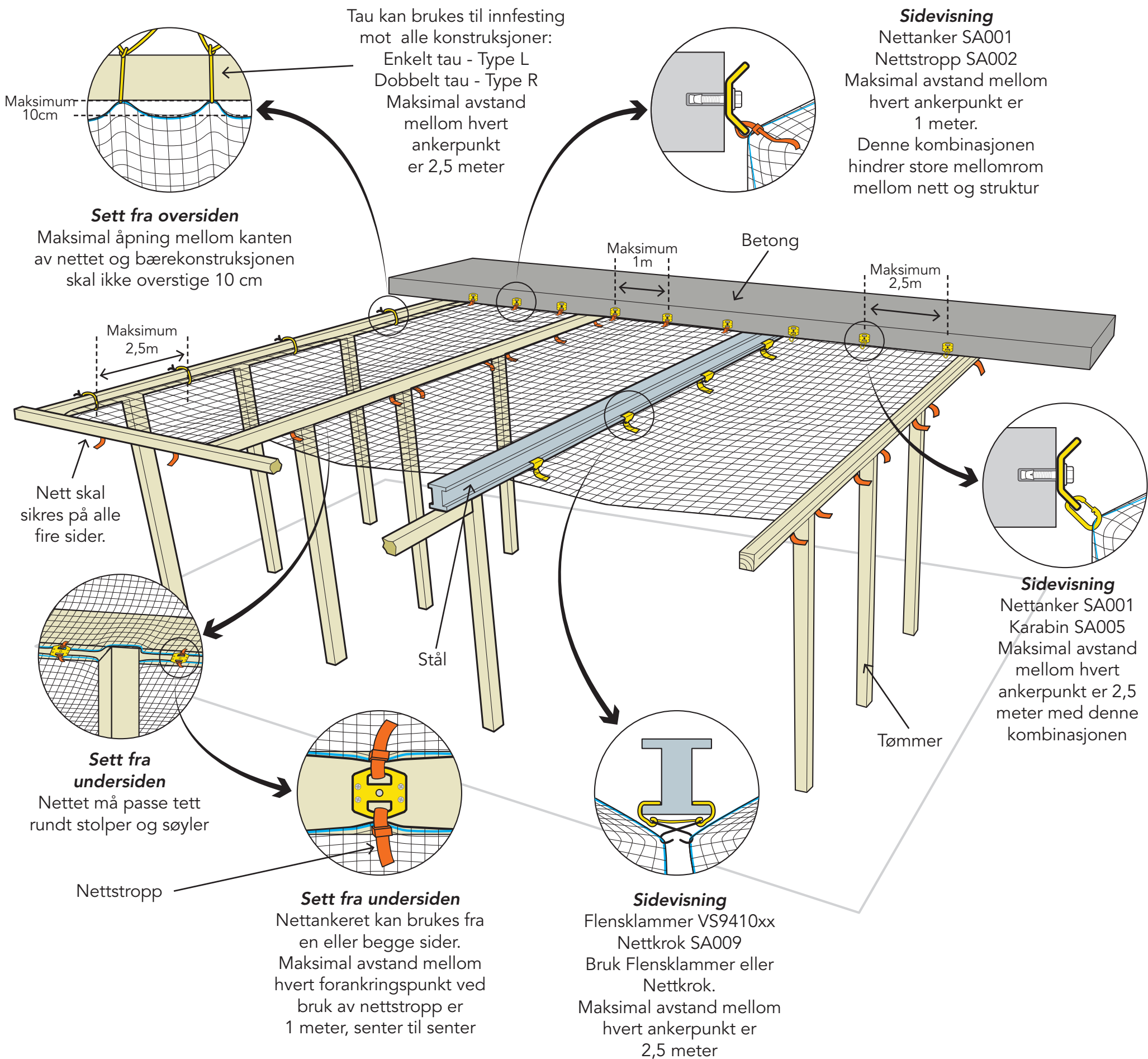
> Figur 1: Montering av nett
