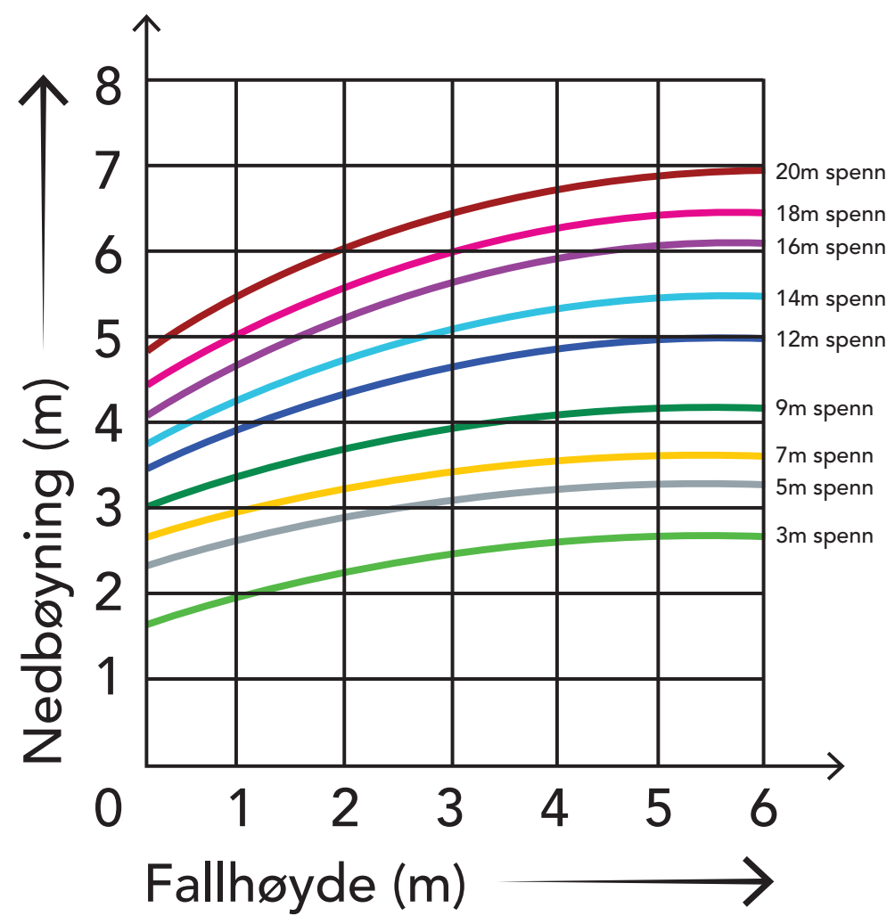
> Figur 7: Nedbøyningsdiagram
