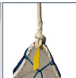
Opphengslinje 3 / 13,5 m SN9001 / 9002 12 mm tau med øye, 30 kN
