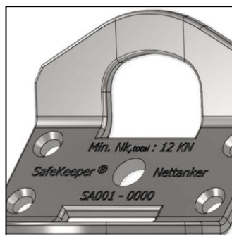
SA001 Nettanker opphengspunkt for montering av nett
