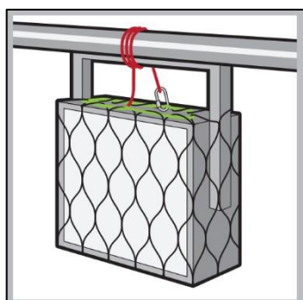
Vaiennett: sikring av fastmontert utstyr.
